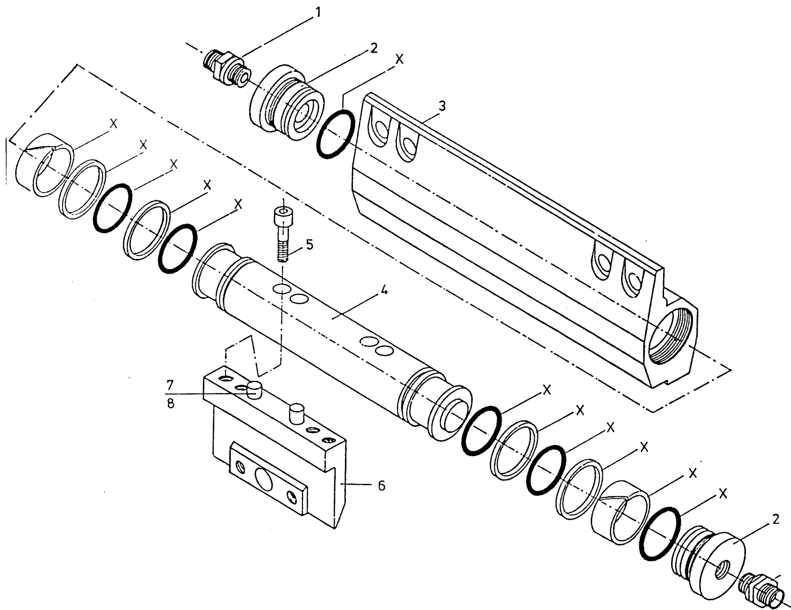
Afb. 10 Achtermescylinder Zylinder Hintermesser
