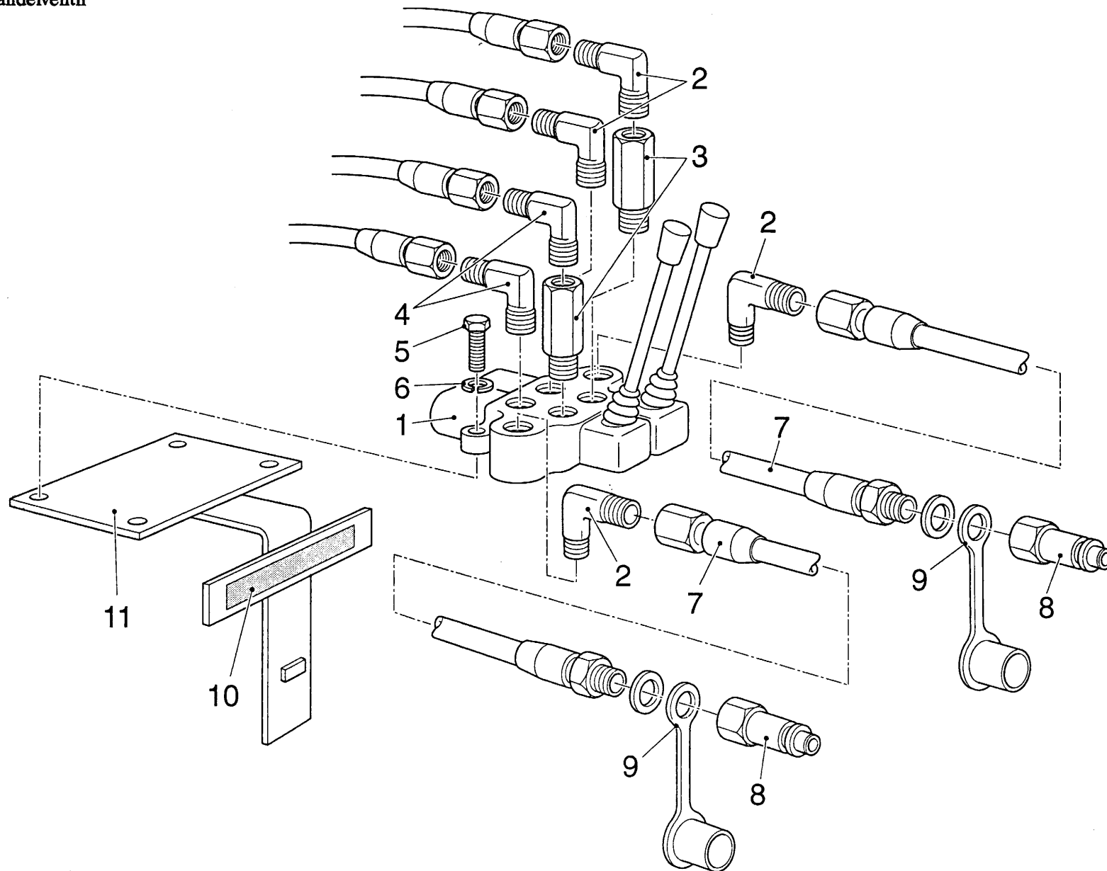
Afb. 8 2-Handelventiel 2-Handelventil
