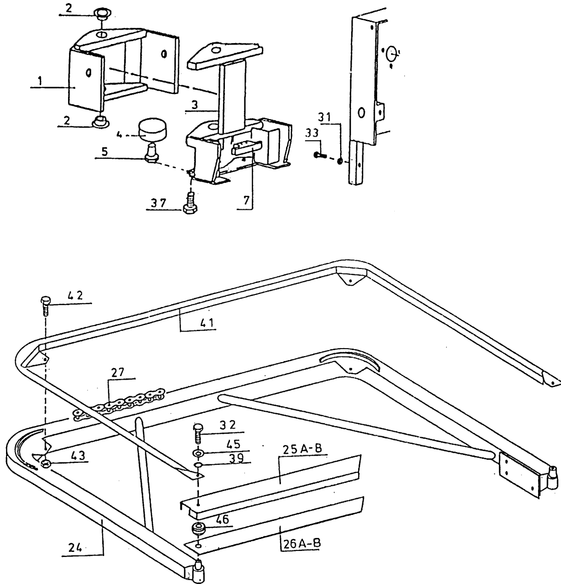
ABB. 3 - FÜHRUNGSRAHMEN, SERIE 06
