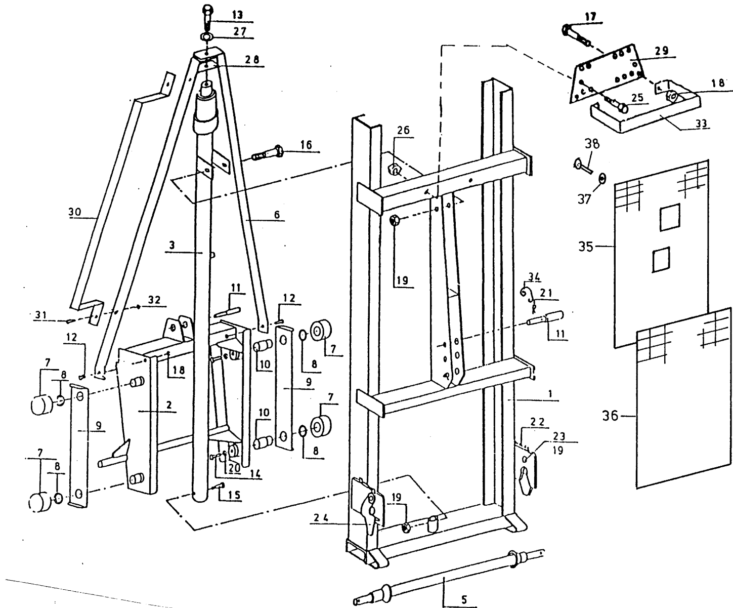
92058/1 ABB. 12 - HUBGERÜST
