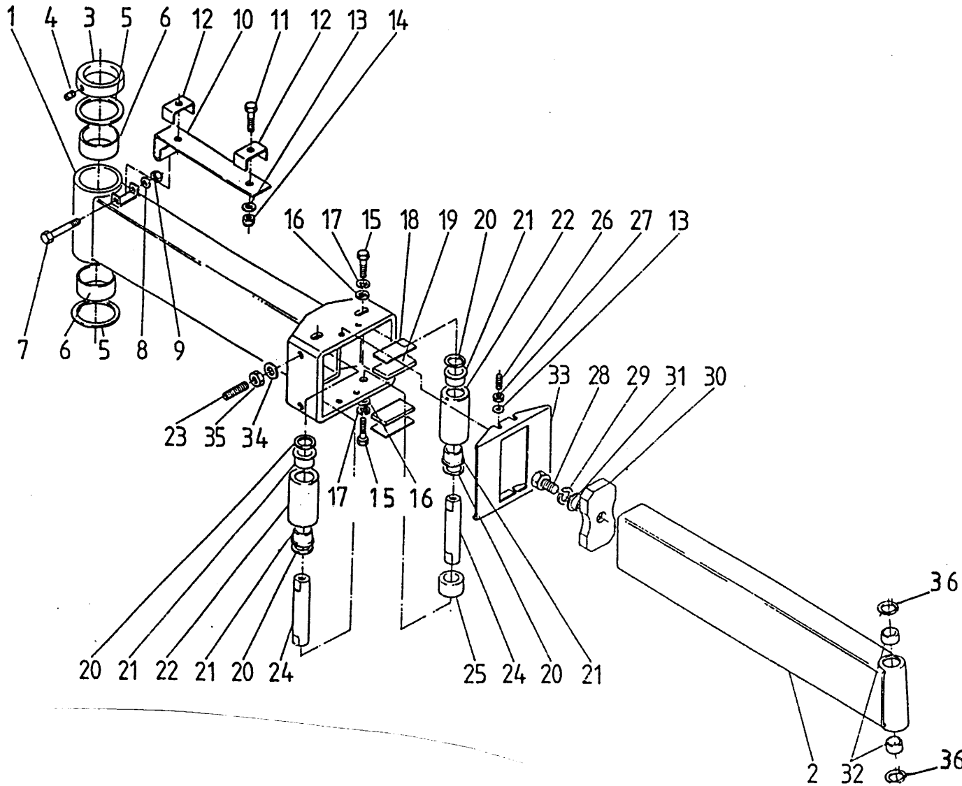
92058/1 ABB. 5 - TELESKOPROHR
